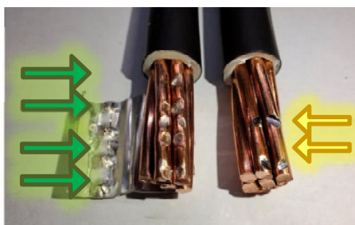
Erhöhung der Kontaktstellen auch innerhalb der VHD-Hülse
